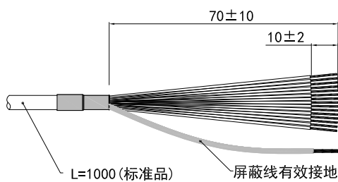
电缆连接
